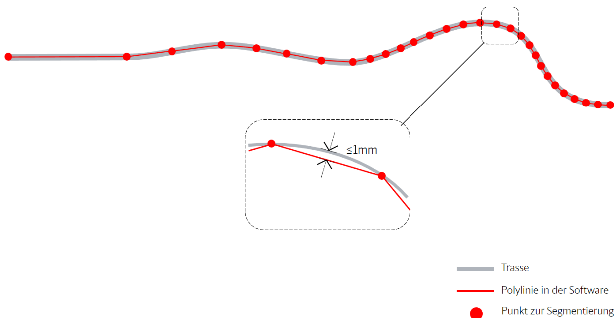
Abbildung 49 Transformation Trassendaten in Polylinie
