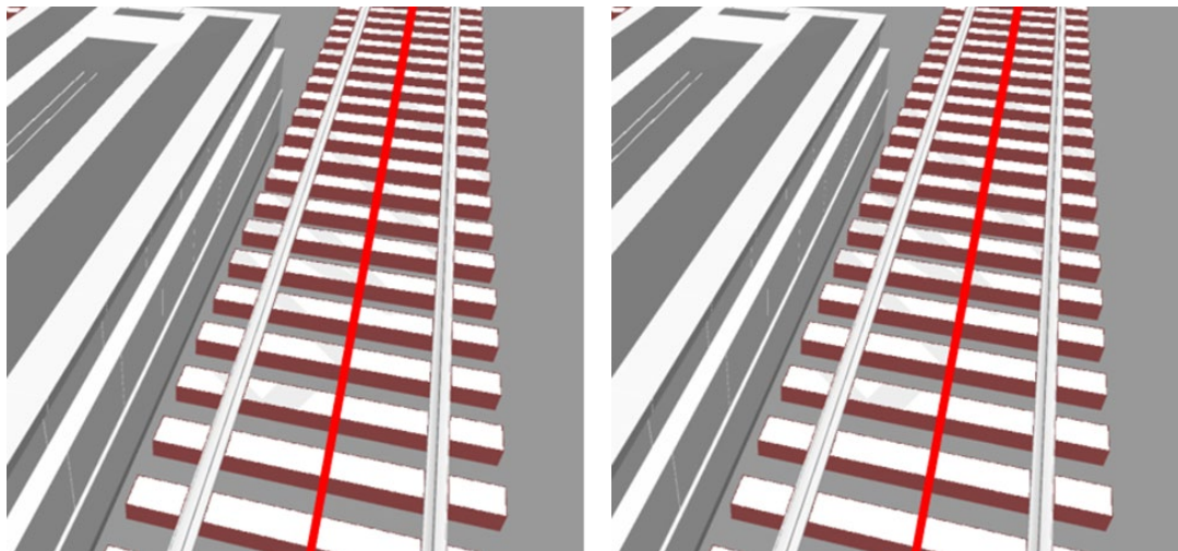
Abbildung 33 Oberbau mit Gleisachse als 3D-Polylinien (links: SOLL, rechts: IST)
