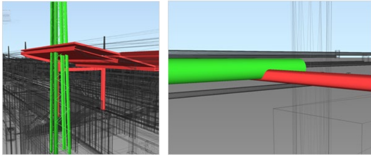
Abbildung 14 Kollisionen der Fachgewerke im Koordinationsmodell
