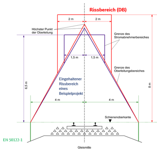
Abbildung 36 Oberleitungsbereich gem. RIL 954.0101A01
