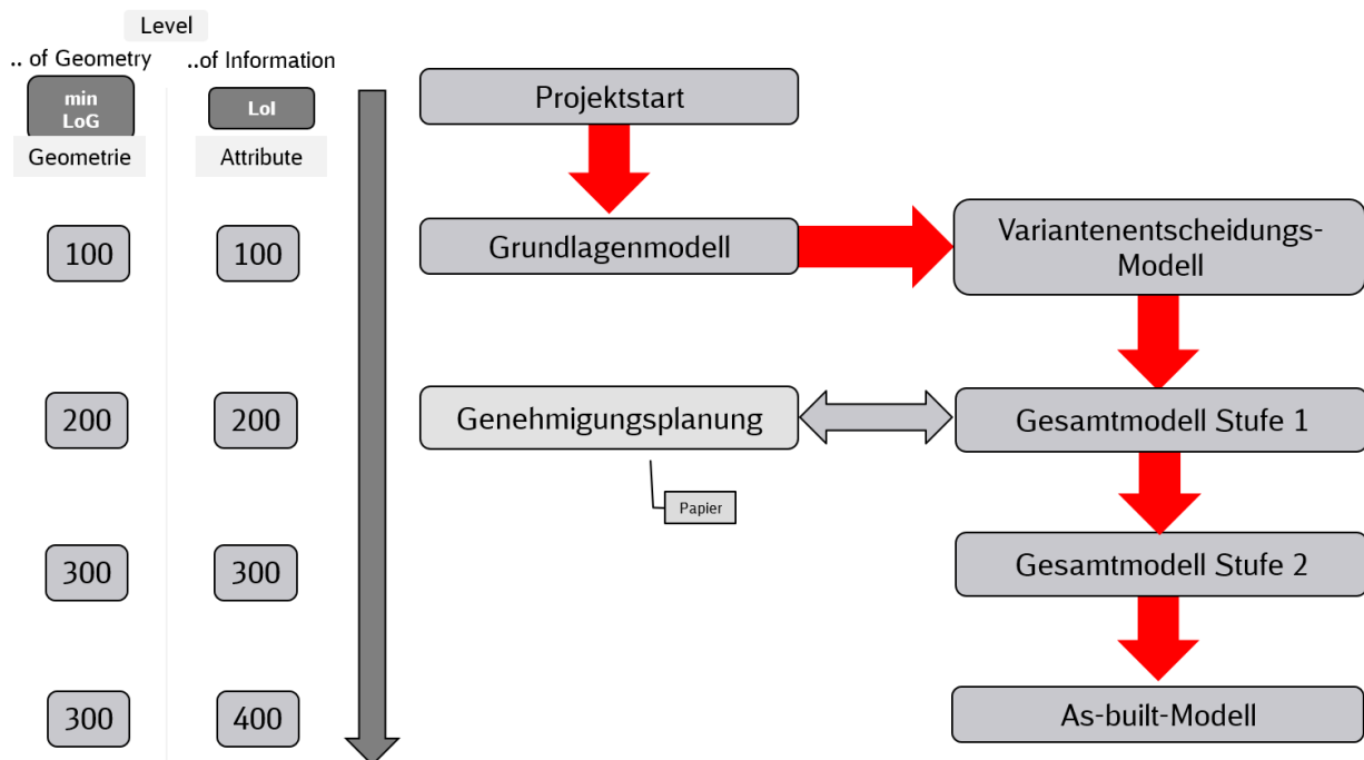
Abbildung 10 Darstellung Planungsablauf mit min. LoG/Lol
