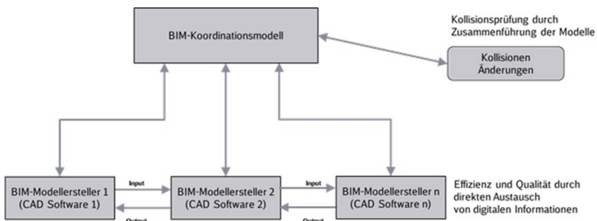
Abbildung 5 Datenaustausch und BIM-Koordinationsmodell
