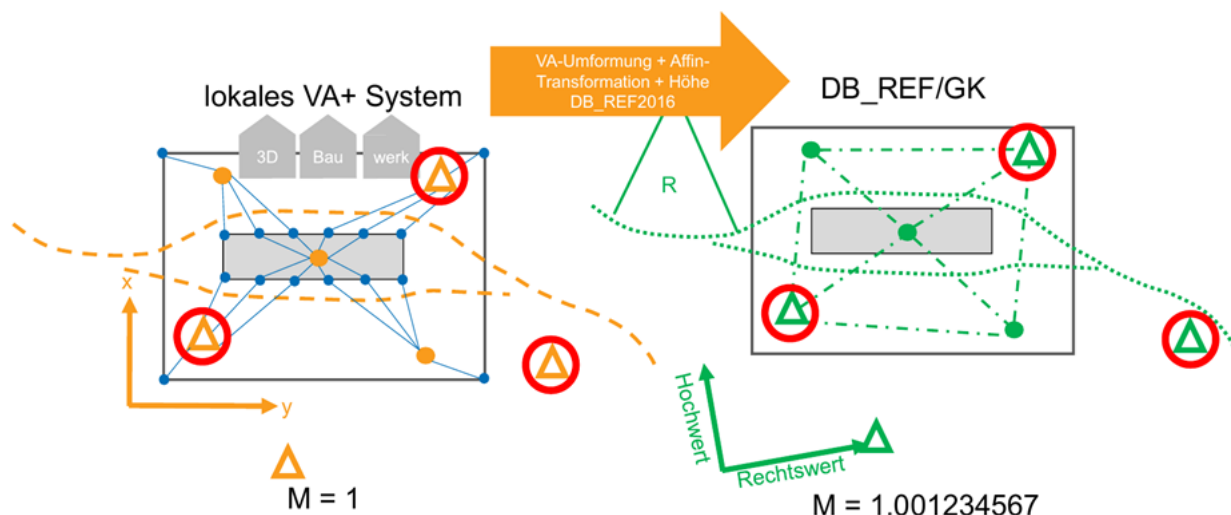
Abbildung 48 DB_REF Netzverdichtung Sonderfall
