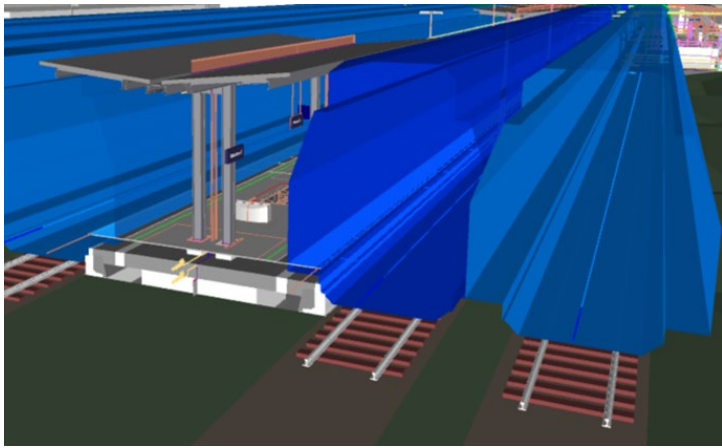
Abbildung 34 Lichtraumprofile an Mittelbahnsteig
