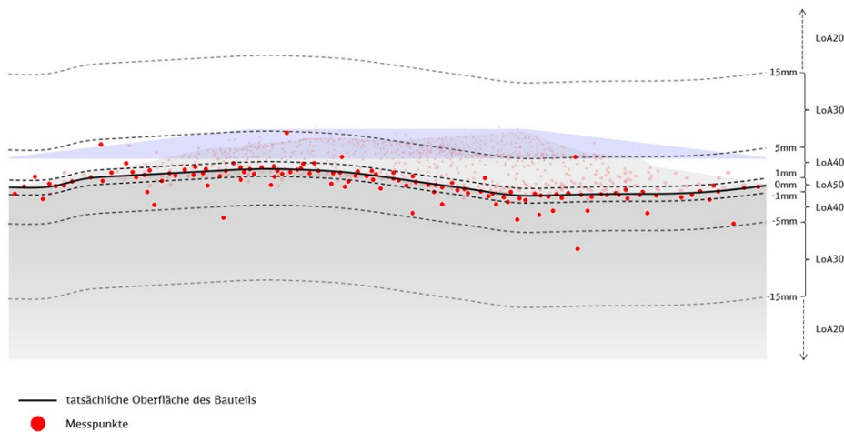
Abbildung 26 Messgenauigkeit Punktwolke
