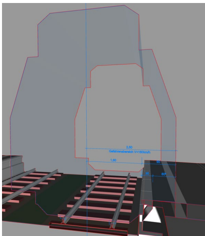
Abbildung 35 Lichtraumprofil inkl. Darstellung Gefahrenbereich
