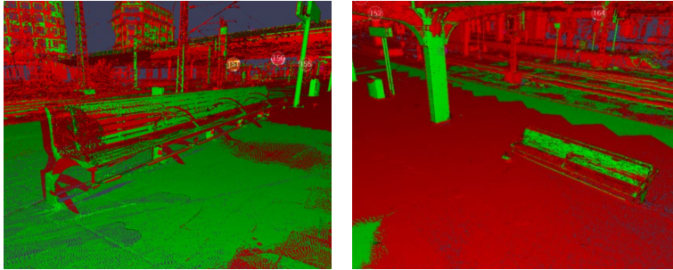
Abbildung 22 Abgleich gebauter IST-Zustands (Punktwolke) mit der Planung (BIM-Modell)*
