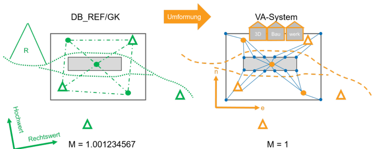
Abbildung 47 Übergeordnete Netzverdichtung Normalfall
