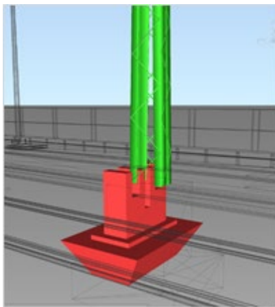
Abbildung 17 Kollision Fundament modularer Bahnsteig mit Mast
