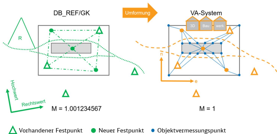
Abbildung 52 Übergeordnete Netzverdichtung Normalfall
