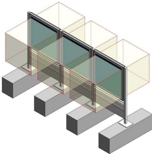
Abbildung 33 Vitrine mit Volumenkörpern als Wartungs- und Instandhaltungsflächen
