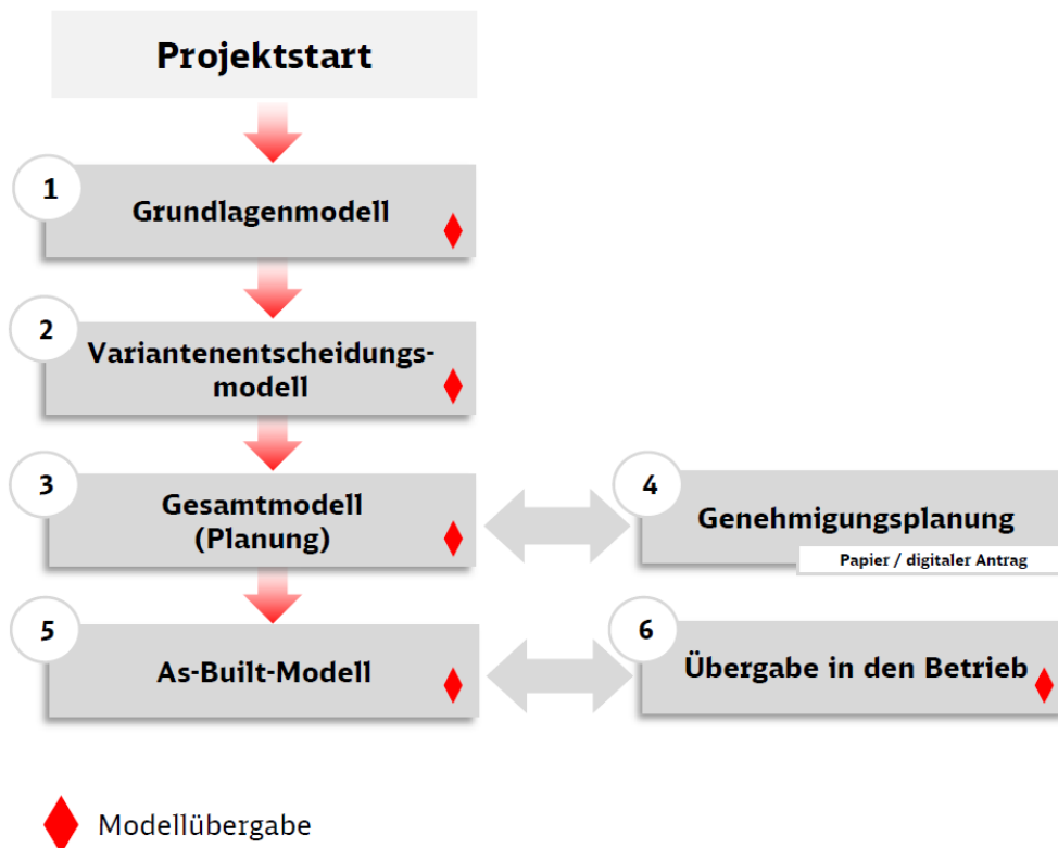
Abbildung 3 BIM-Projektablauf auf Modellebene (Prinzipskizze)
