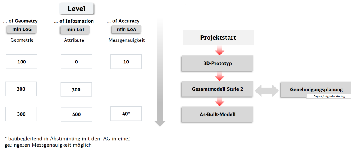
Abbildung 10 Darstellung Planungsablauf mit min. LoG/LoI/LoA für die EinfachBIM Projekte
